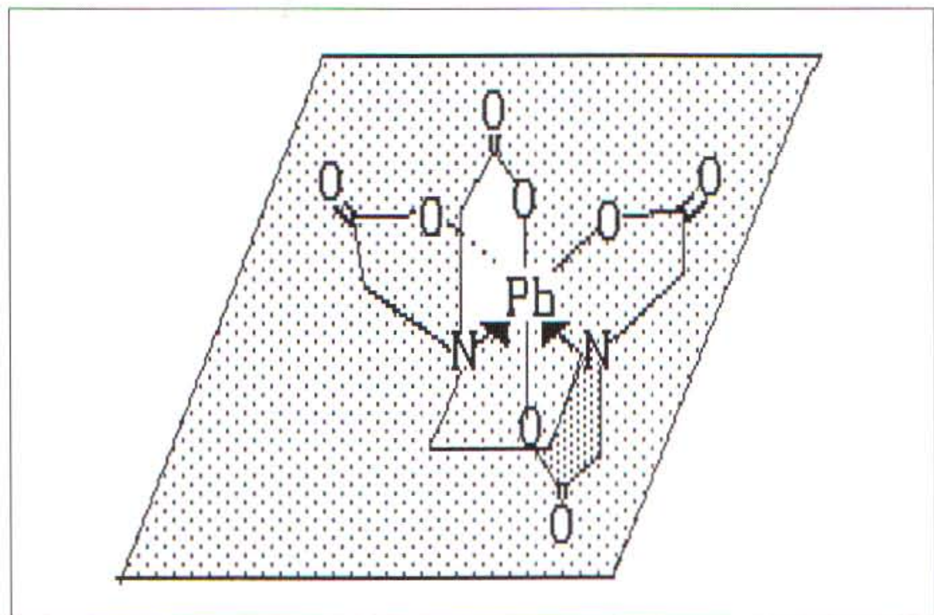
Fig 3. Kelatdannelse mellom EDTA og bly. Bly blir inkorporert i 5 heterocykliske ringer. (Modifisert tegning fra Meyers FH, Jawets E, Goldfien A. A Review of Medical Pharmacology , 7th ed. Lange, 1980). Jevnfør med Fig 4.
